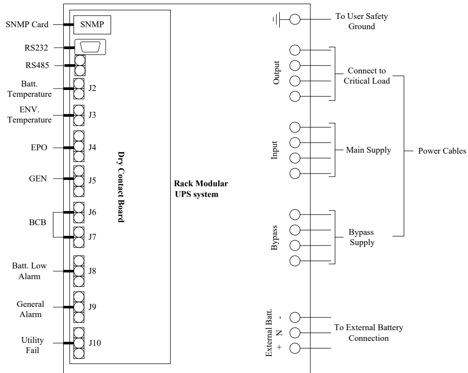
Fig. 4-1: Schema circuito
