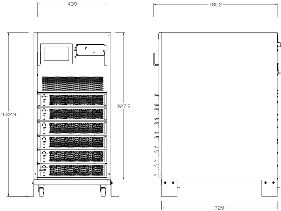
Fig. 4-6: Dimensioni esterne UPS a sei moduli
