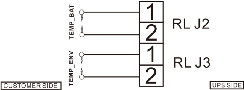
Fig. 1-7: Schema interfacce J2 e J3
