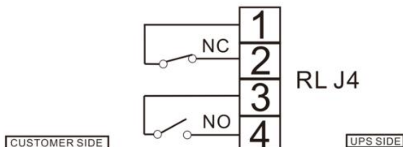
Fig. 1-8: Schema di collegamento per EPO remoto
