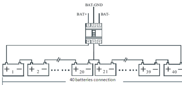
Fig. 2-1: Schema collegamento batterie
