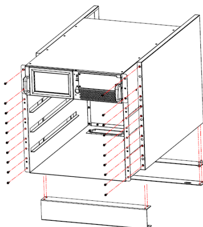
(a) Rimuovere i pannelli laterali e i supporti
