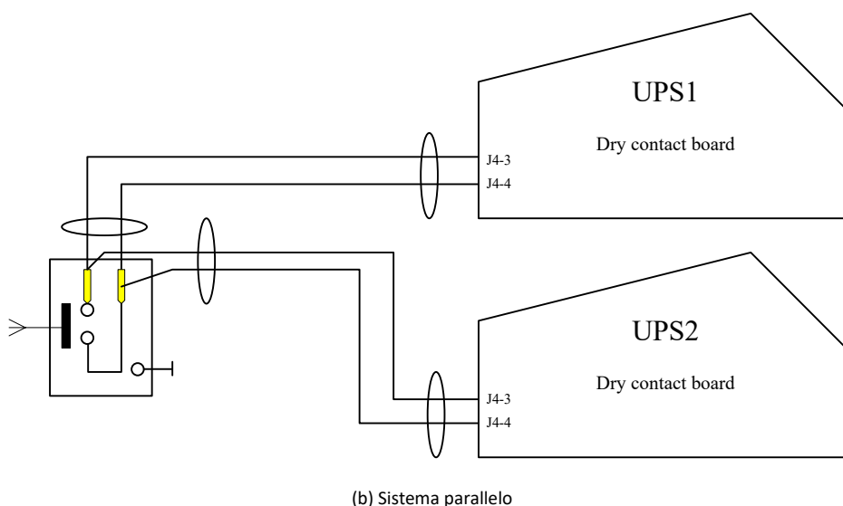
Fig. 3-1: Schema del circuito dell'EPO
