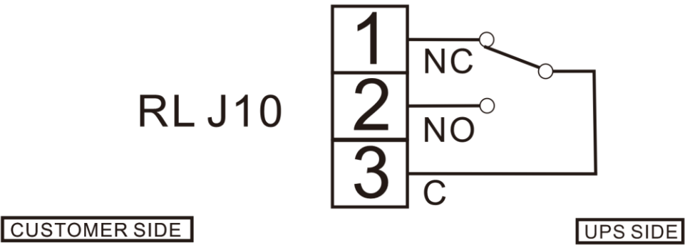
Fig. 1-13: Schema collegamento contatto mancanza rete
