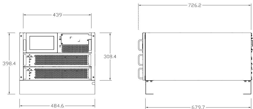
Fig. 4-3: Dimensioni esterne dell'UPS a due moduli
