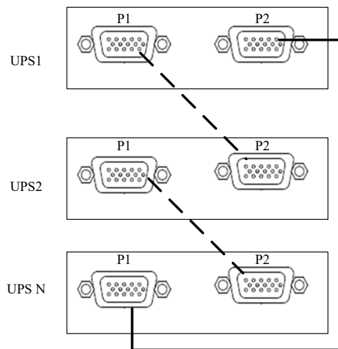
Fig. 8-3: Collegamento dei cavi di parallelo del sistema "1+N"
