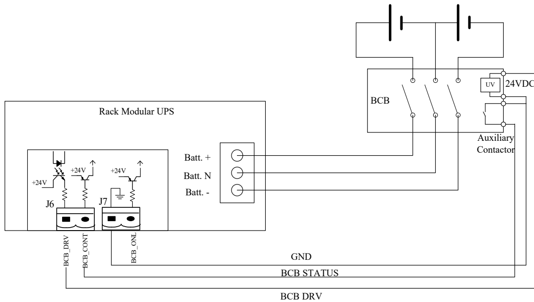
Fig. 4-2: Collegamento batterie esterne
