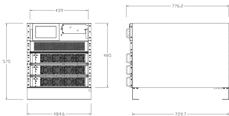
Fig. 4-4: Dimensioni esterne UPS a tre moduli
