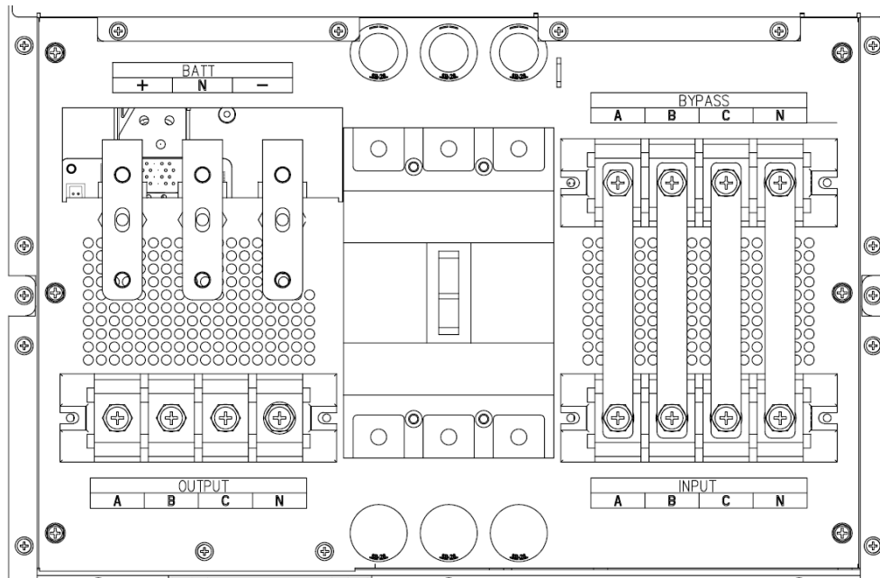
(c) Connessione 60KVA/90KVA
