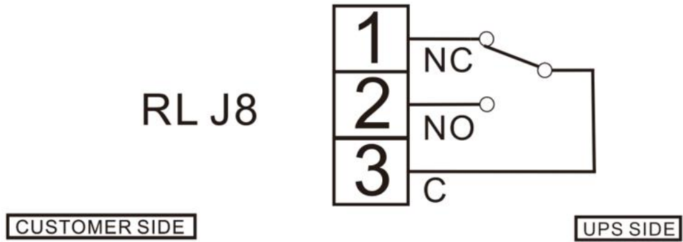
Fig. 1-11: Schema di collegamento contatto allarme batteria
