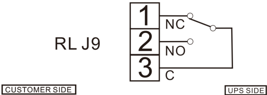
Fig. 1-12: Schema di collegamento contatto pulito allarme generale
