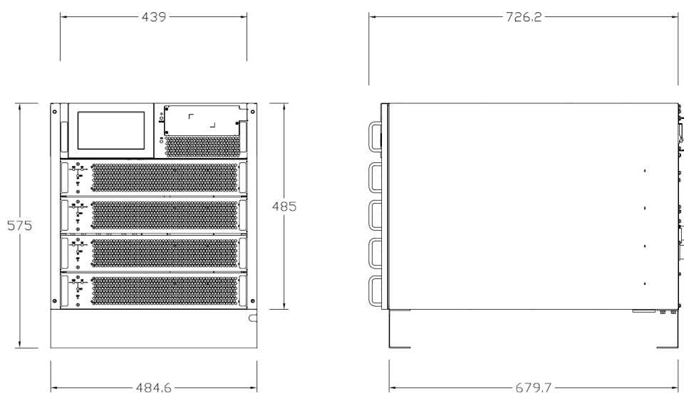
Fig. 4-5: Dimensioni esterne UPS a quattro moduli
