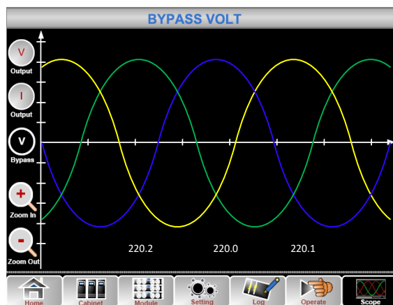
Fig. 7-12: forma d'onda di uscita e bypass
