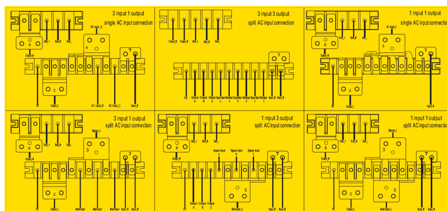
Fig. A-1: Connessione sistema modulare sistema a 2 e 4 moduli
