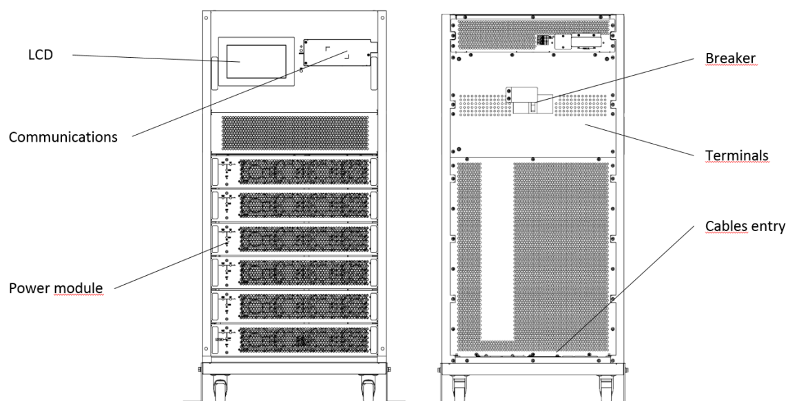
(d) Cabinet a 6 moduli
