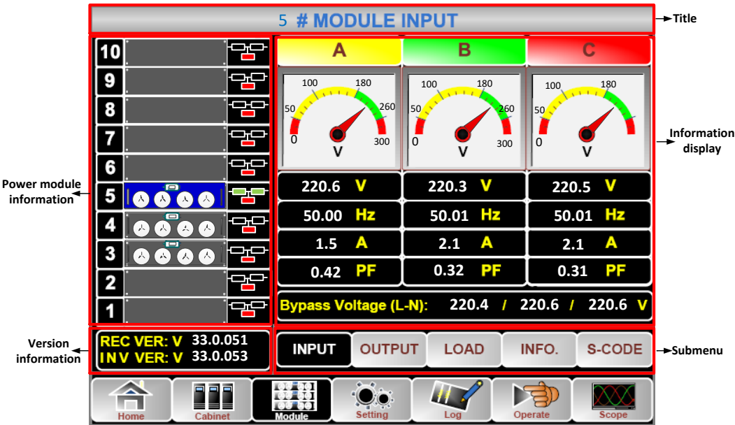
Fig. 7-7: Informazioni modulo di potenza
