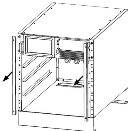
(a) Rimuovere le cornici metalliche decorative laterali
