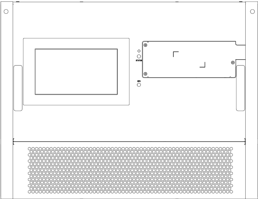
(d) Modulo bypass 90kVA
