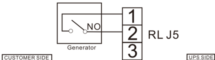
Fig. 1-9: Connessione del generatore
