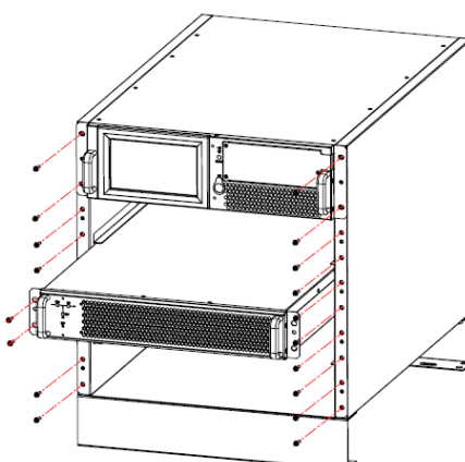
(b) Inserire modulo di potenza
