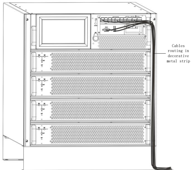
Fig. 4-12: Percorso cavi (contatti puliti, RS485, SNMP)
