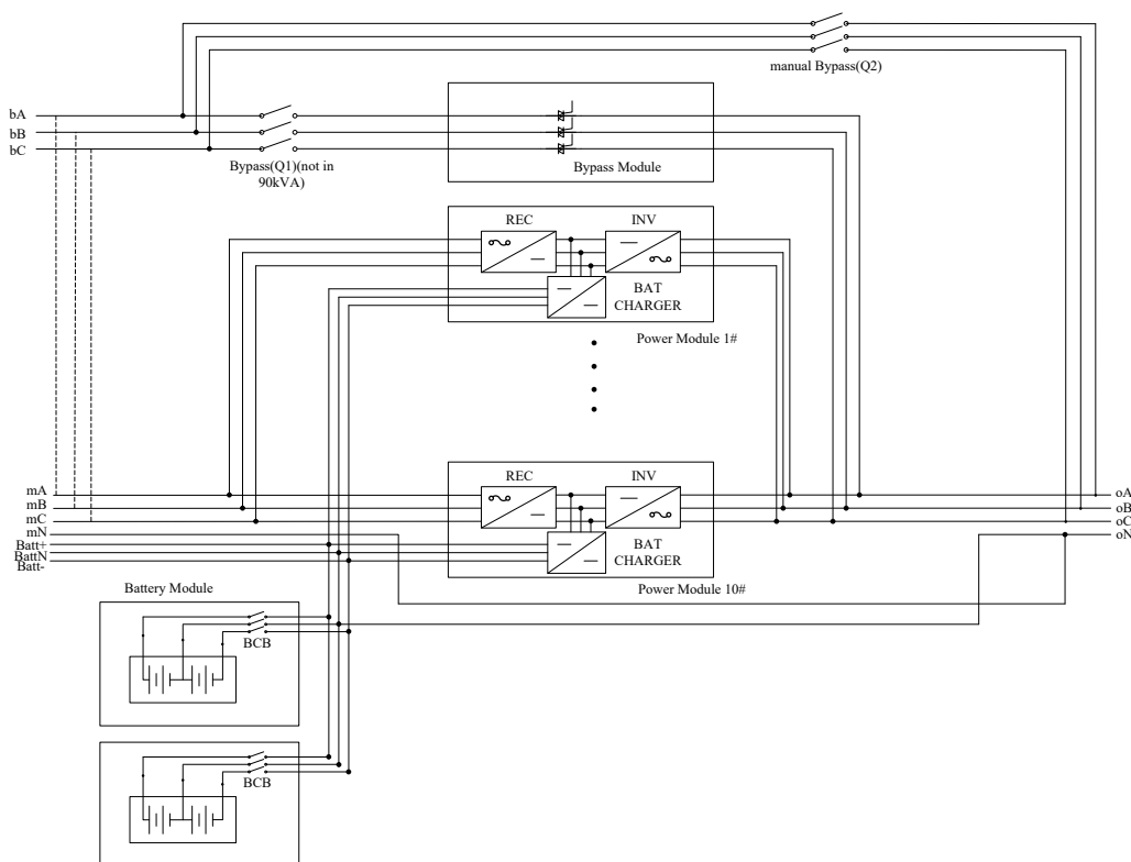
Fig. 5-1: Schema unità singola
