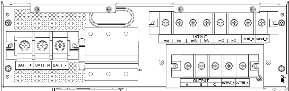
(b) Connessione 30KVA/45KVA
