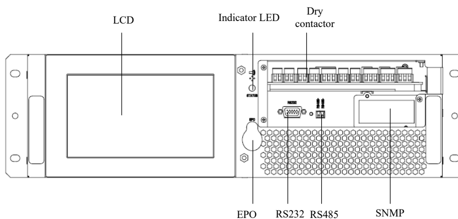
(a) Modulo bypass 20kVA/40kVA
