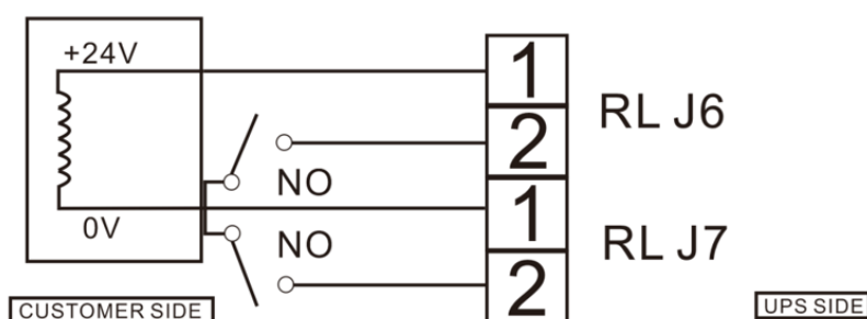
Fig. 1-10: Interfaccia interruttori di batteria
