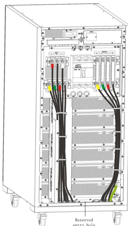
(b) Ingresso cavi di un cabinet a 6 moduli
