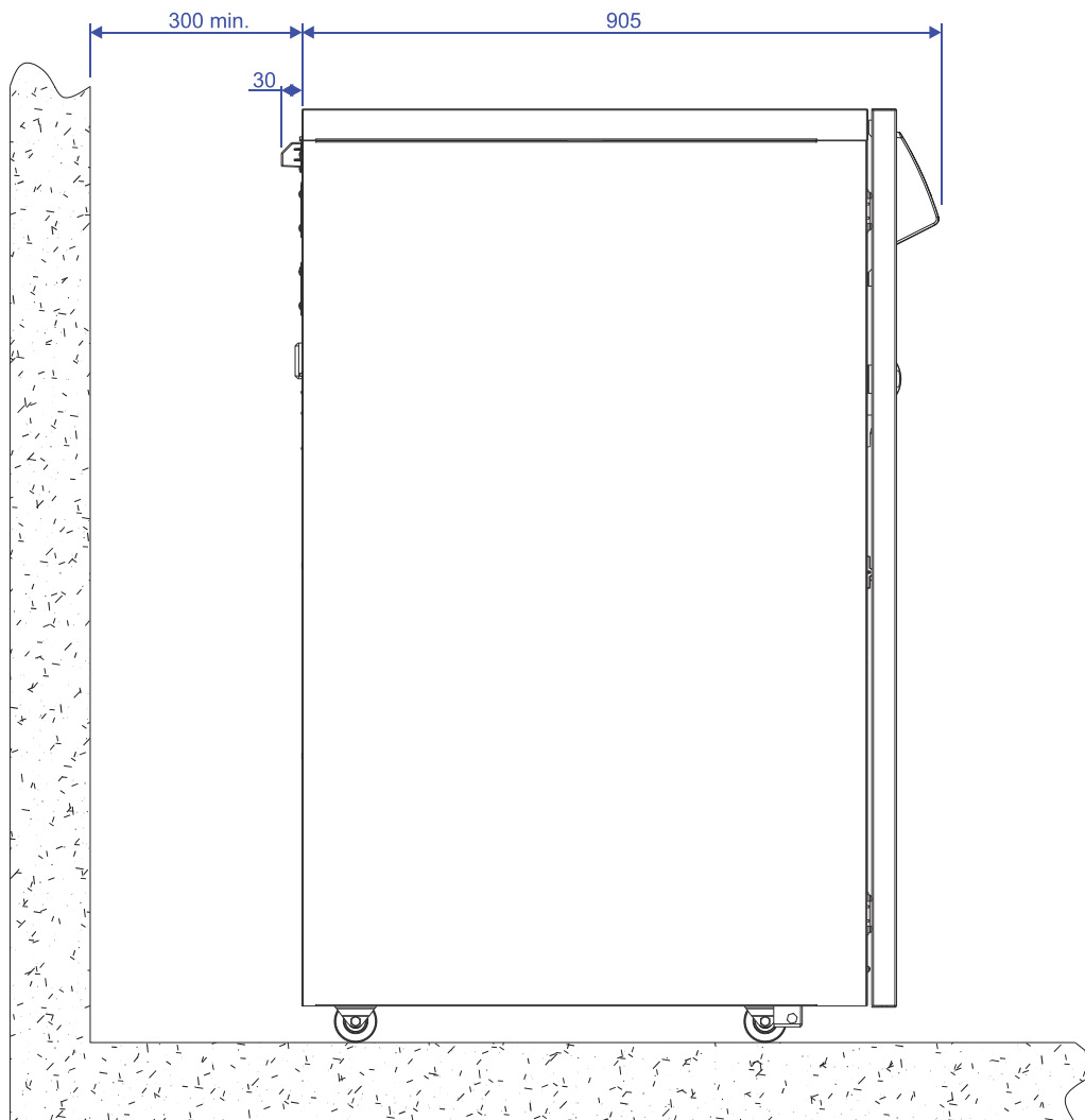
VISTA LATERALE
