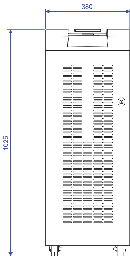
VISTA FRONTALE
