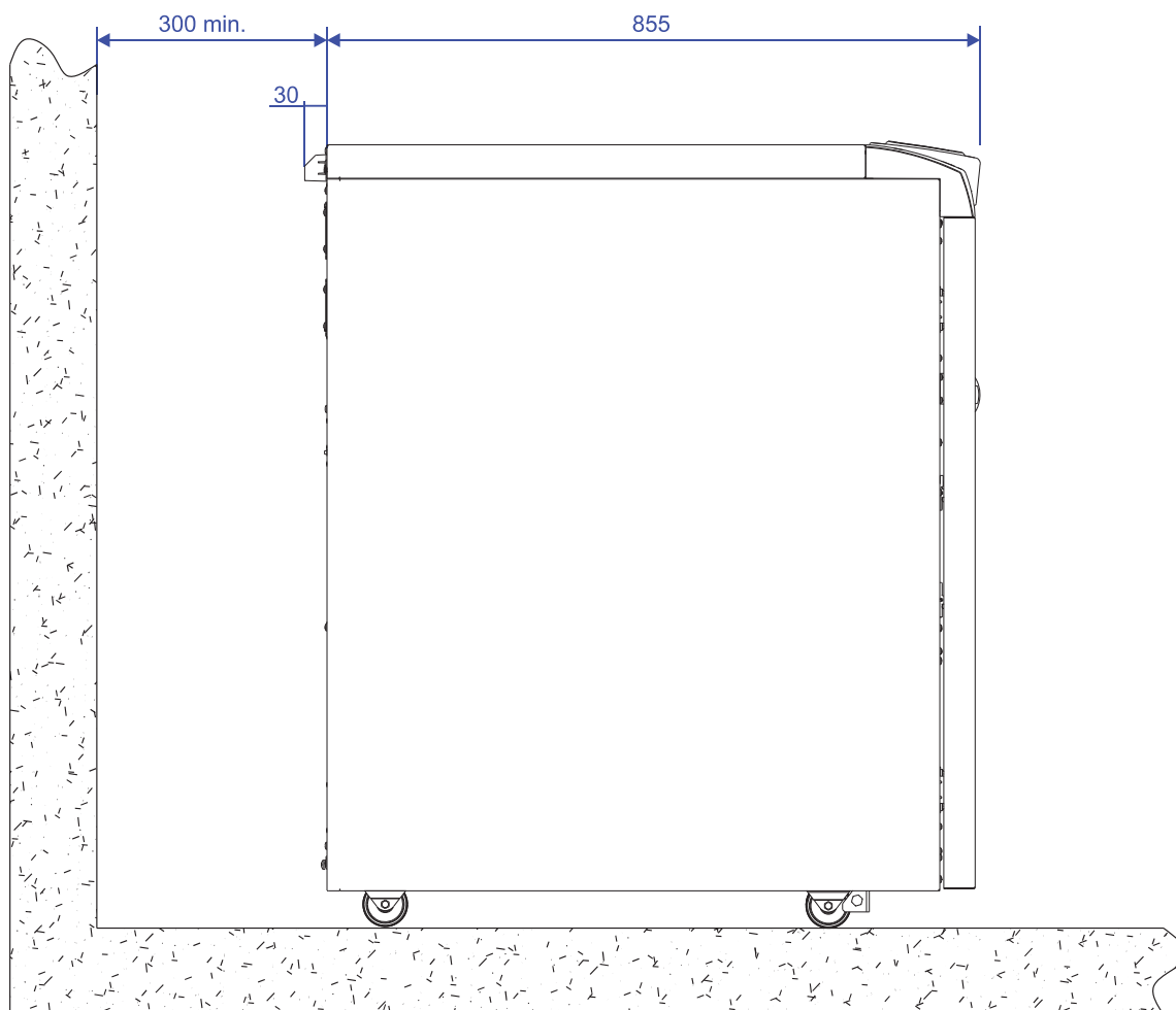
VISTA LATERALE
