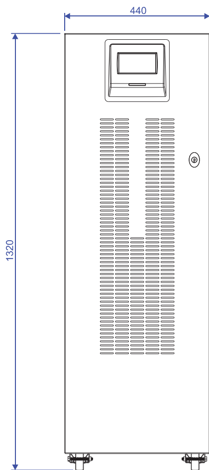
VISTA FRONTALE
