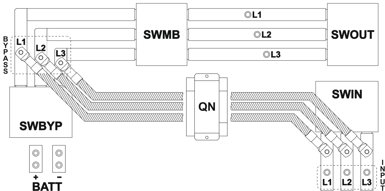
125KVA - BYPASS-ANSCHLUSS AN EINGANGSLEITUNG
