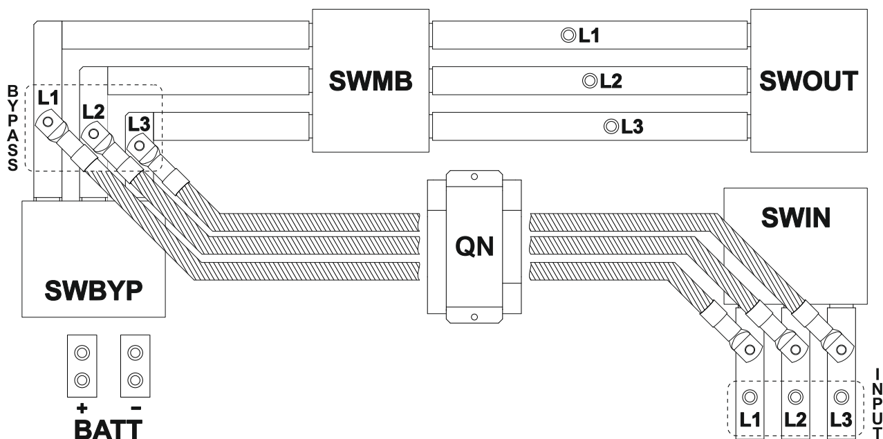
125KVA - BYPASS COLLEGATO ALLA LINEA DI INGRESSO
