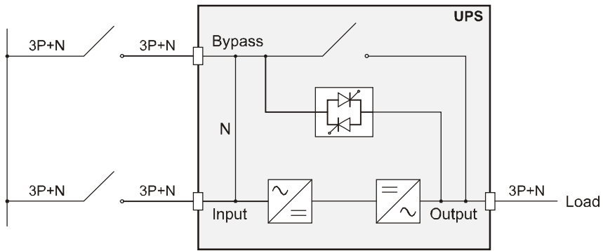
SAI sin variación de régimen de neutro y con entrada bypass separado.
