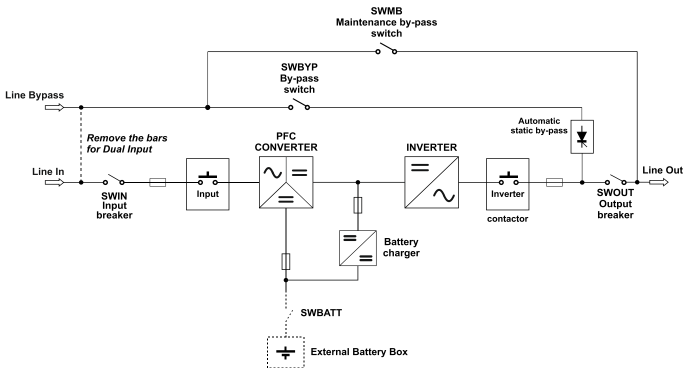
Schéma fonctionnel de l'UPS
