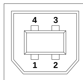
CONNECTEUR USB
