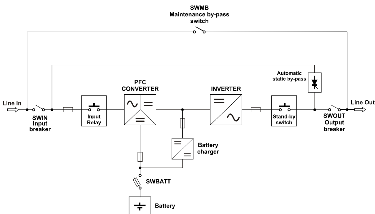
Schéma des connexions de l'Onduleur
