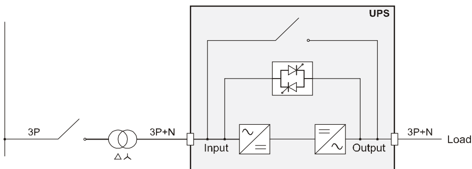
UPS con isolamento galvanico in ingresso
