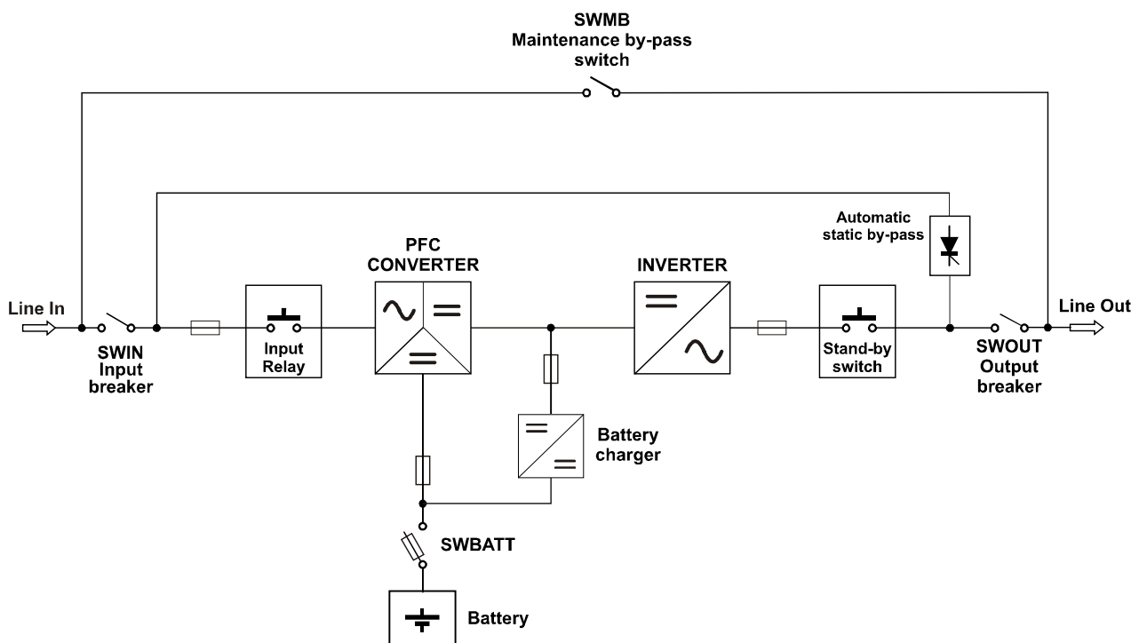
Diagramma a blocchi dell'UPS
