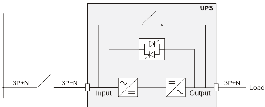
UPS senza variazione di regime di neutro
