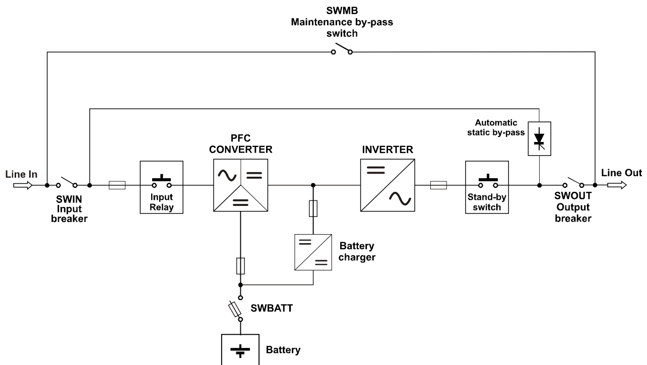
Diagrama de bloques del SAI
