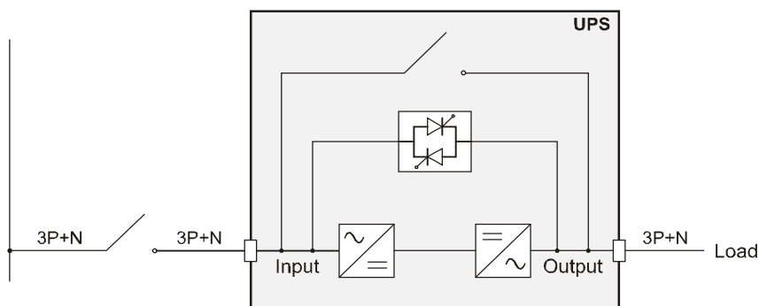
SAI sin variación de régimen de neutro
