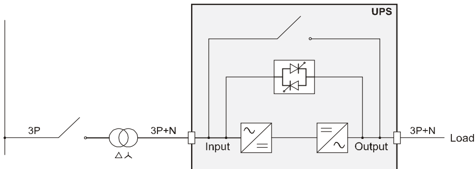
SAI con aislamiento galvánico en entrada
