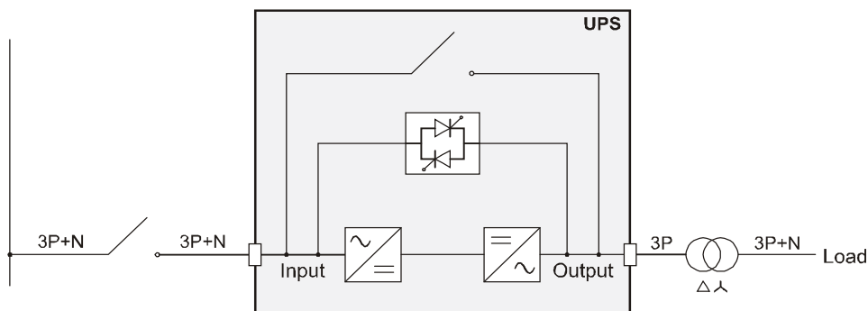
UPS con isolamento galvanico in uscita
