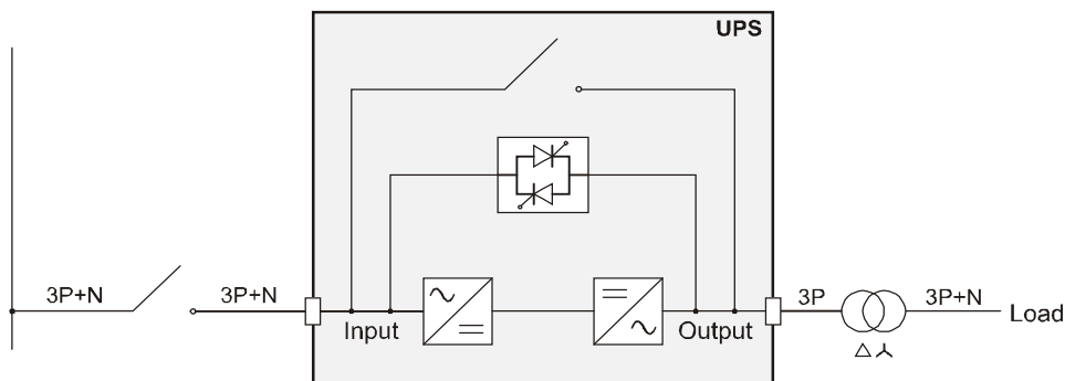
SAI con aislamiento galvánico en salida
