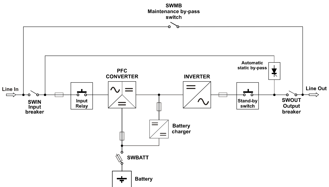
Blockschaema der USV
