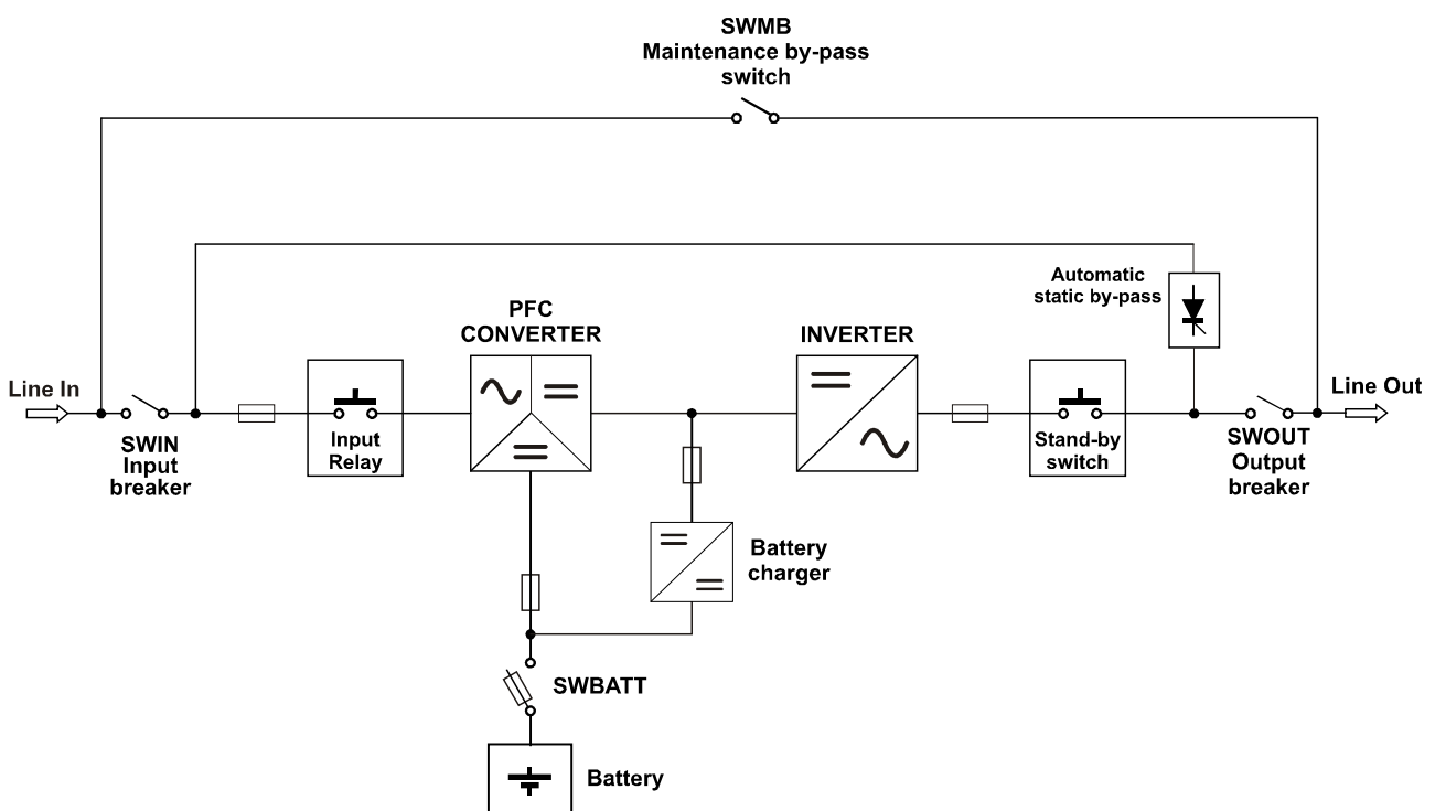
Blockschema der USV
