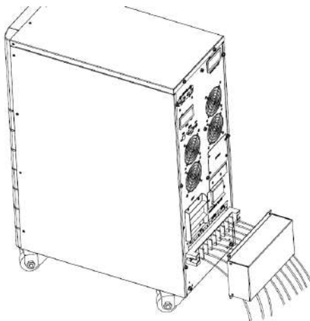
(a) Ingresso cavi
