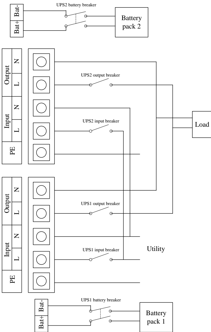
(a) Schema di connessione UPS da 6 e 10kVA
