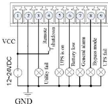
Fig.7 Schema collegamento scheda contatti
