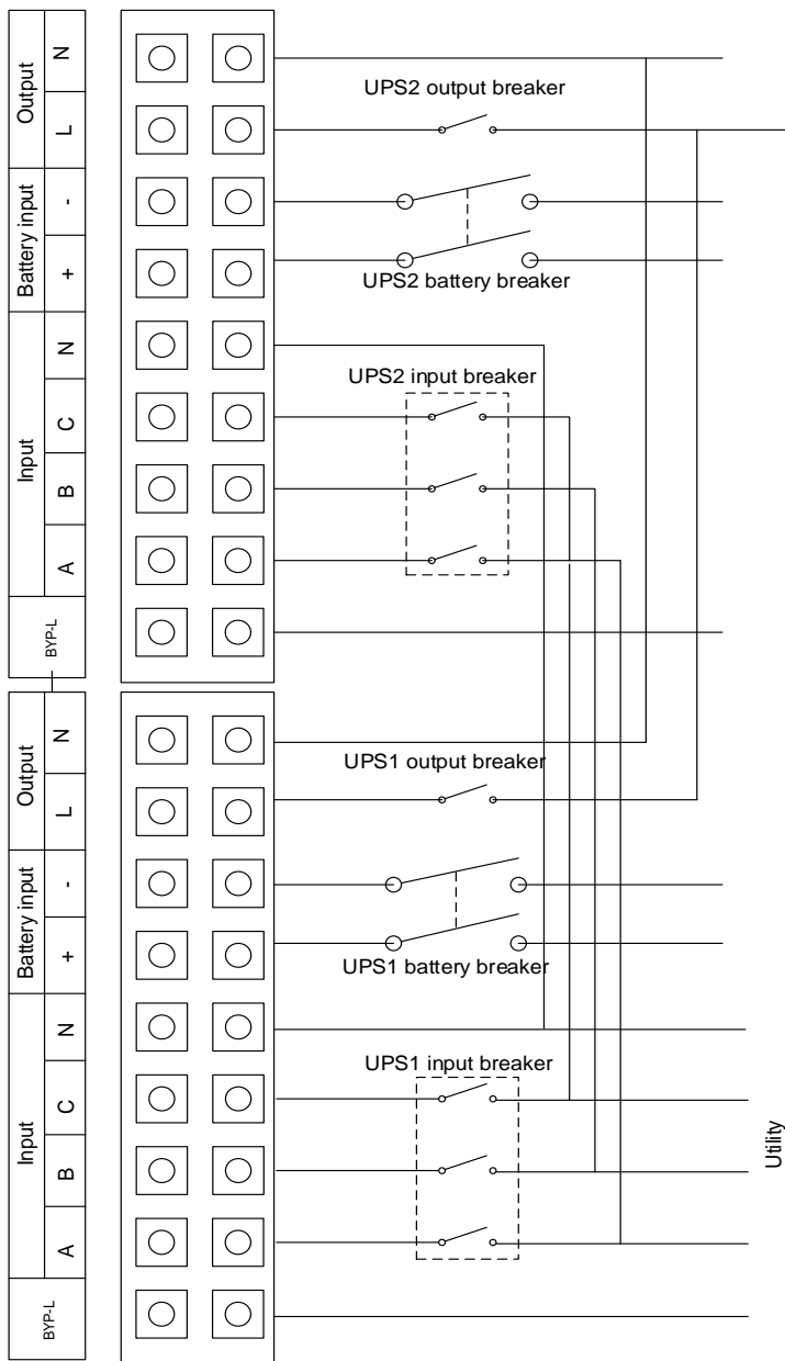
Fig.6 Schema di collegamento 20kVA-KS
