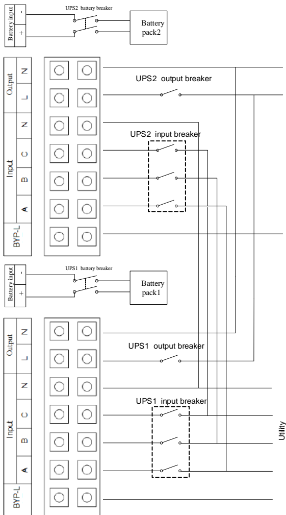
Fig.5 Schema di collegamento 10kVA-KS
