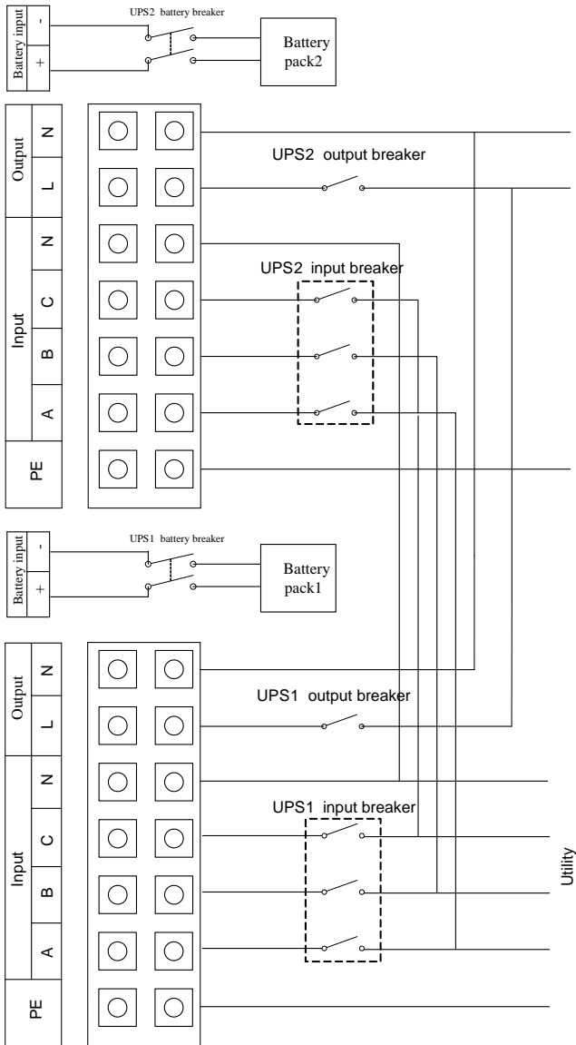
Fig.5 Schéma de câblage pour mise en parallèle ZY120-10K-31-KS
