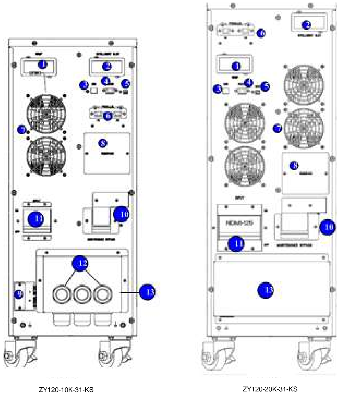
Fig 2. Vue arrière des UPS
