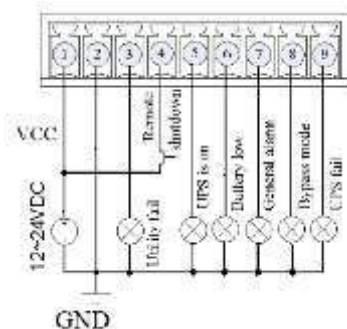
(a) Contatti tipo Phoenix
