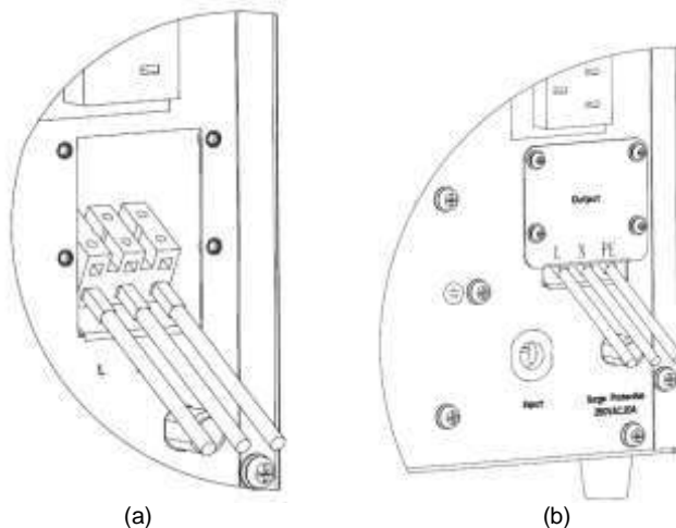
Fig.3 Morsetti di uscita del 3KVA
